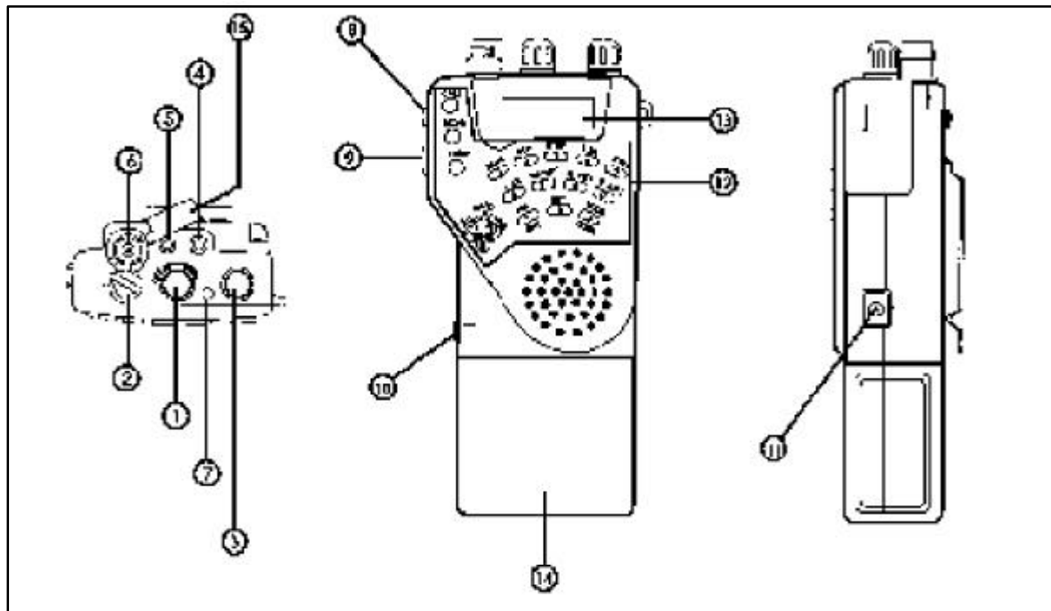
Abb. Bedienelemente und Anschlüsse
